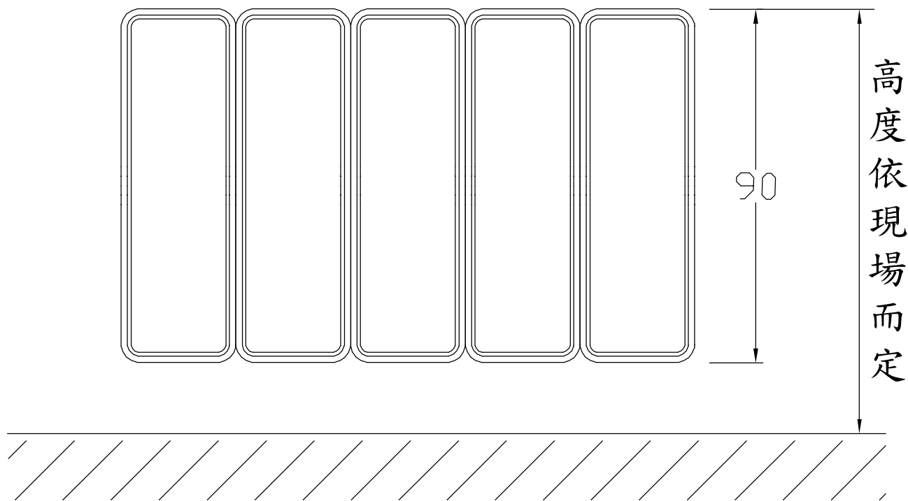
柱角防撞條施工位置圖
