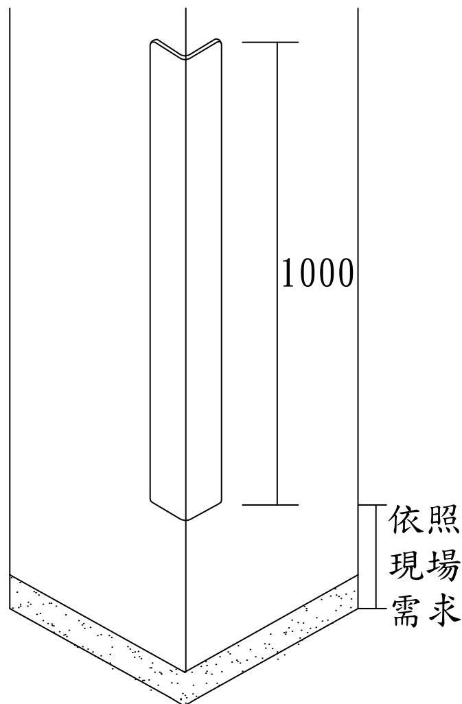
柱角防護條施工位置圖
