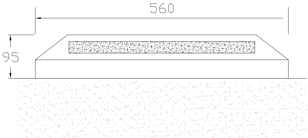
正立面圖
