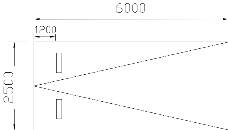
施工位置圖
