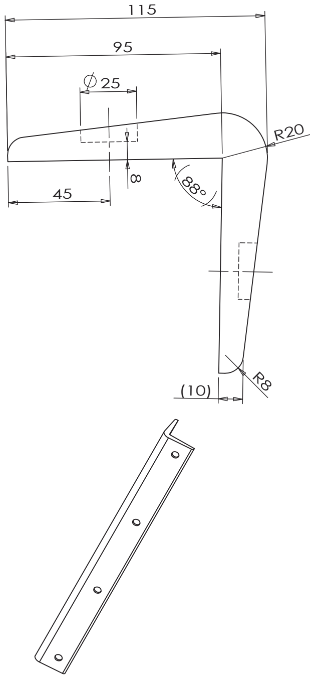
防撞條平面示意圖
