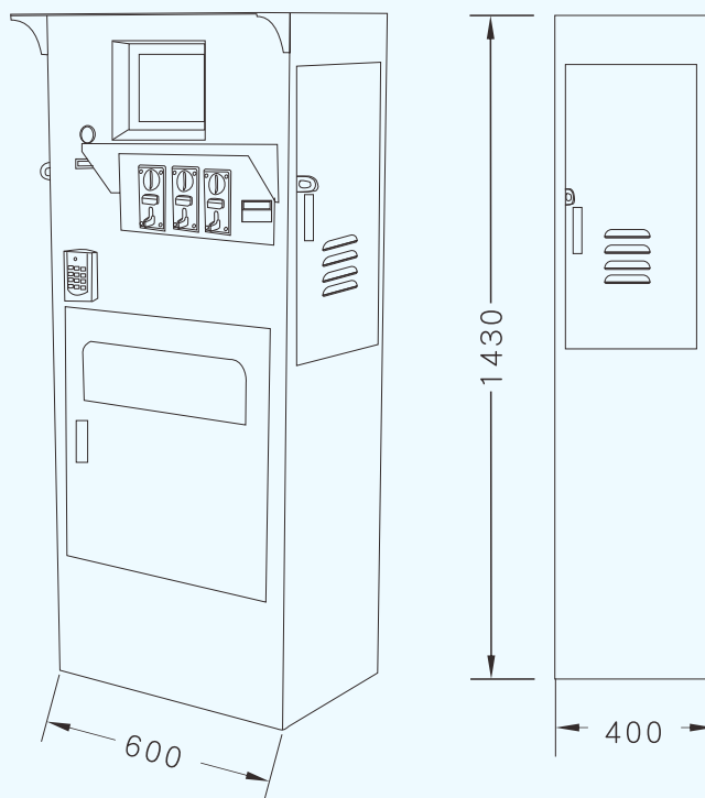
正視圖
