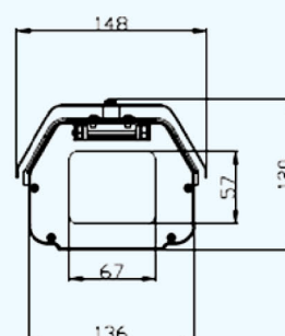
正視圖
